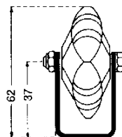
Rolle montiert in oberer Lochreihe Wheel mounted in upper hole
