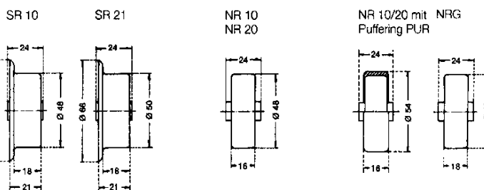
Abmessungen Röllchen Dimension wheels
